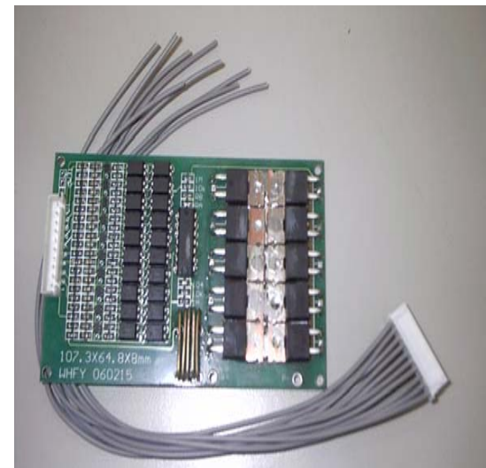
13S 50A Protection Module
